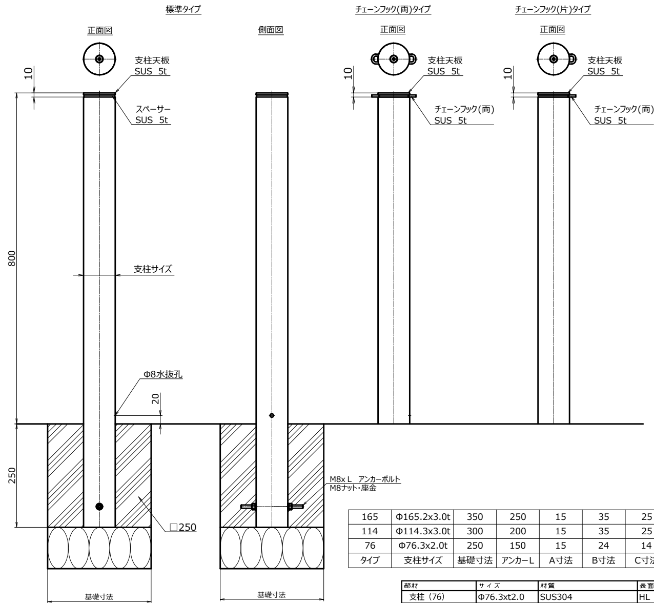
基本図(S=1/6)
