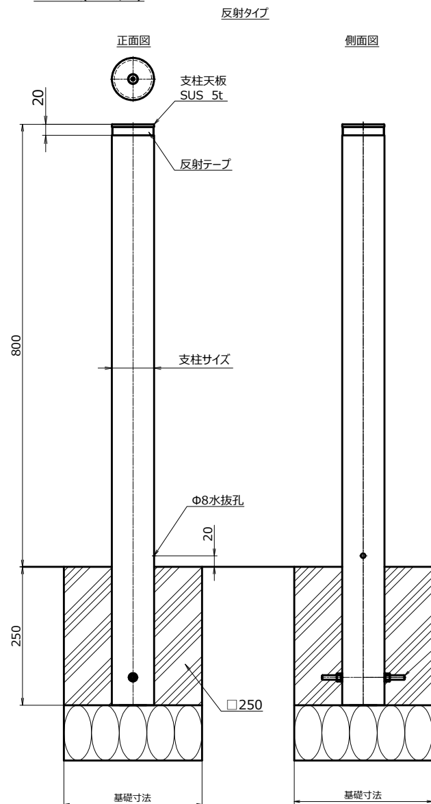
基本図(S=1/6)
