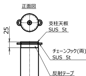
チェーンフック(両)タイプ
