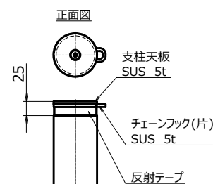
チェーンフック(片)タイプ
