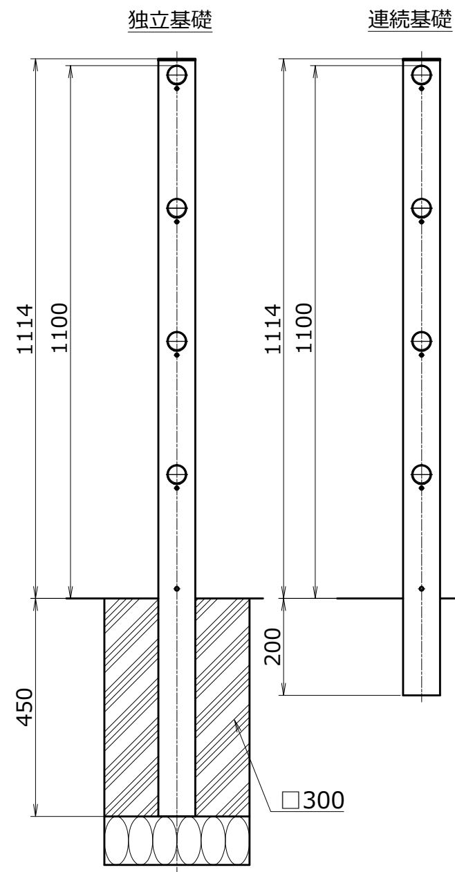
側面図 S=1/10
