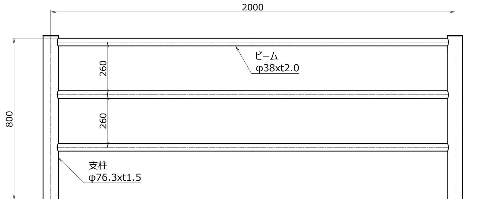
正面図 S=1/10
