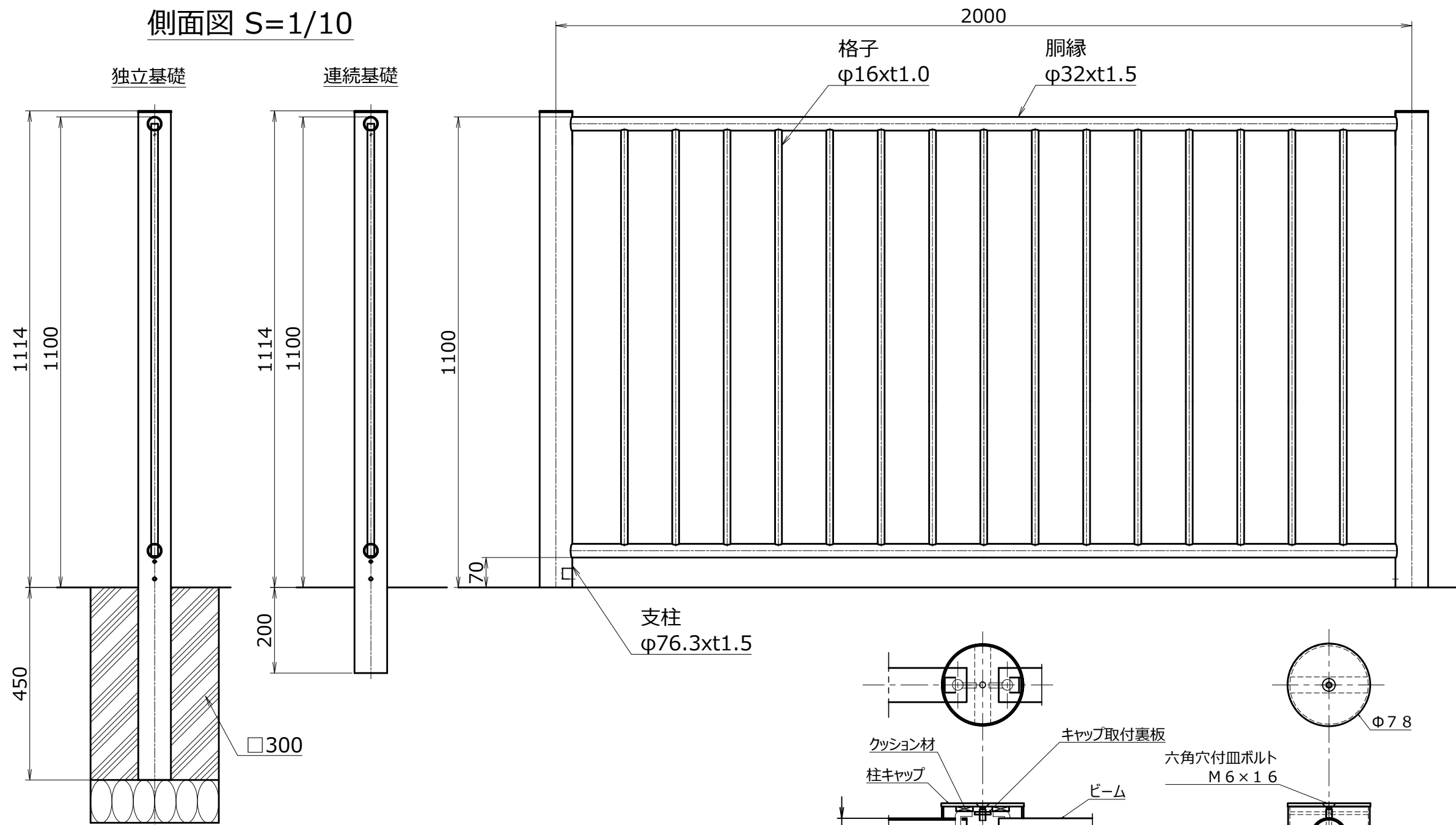
正面図 S=1/10
