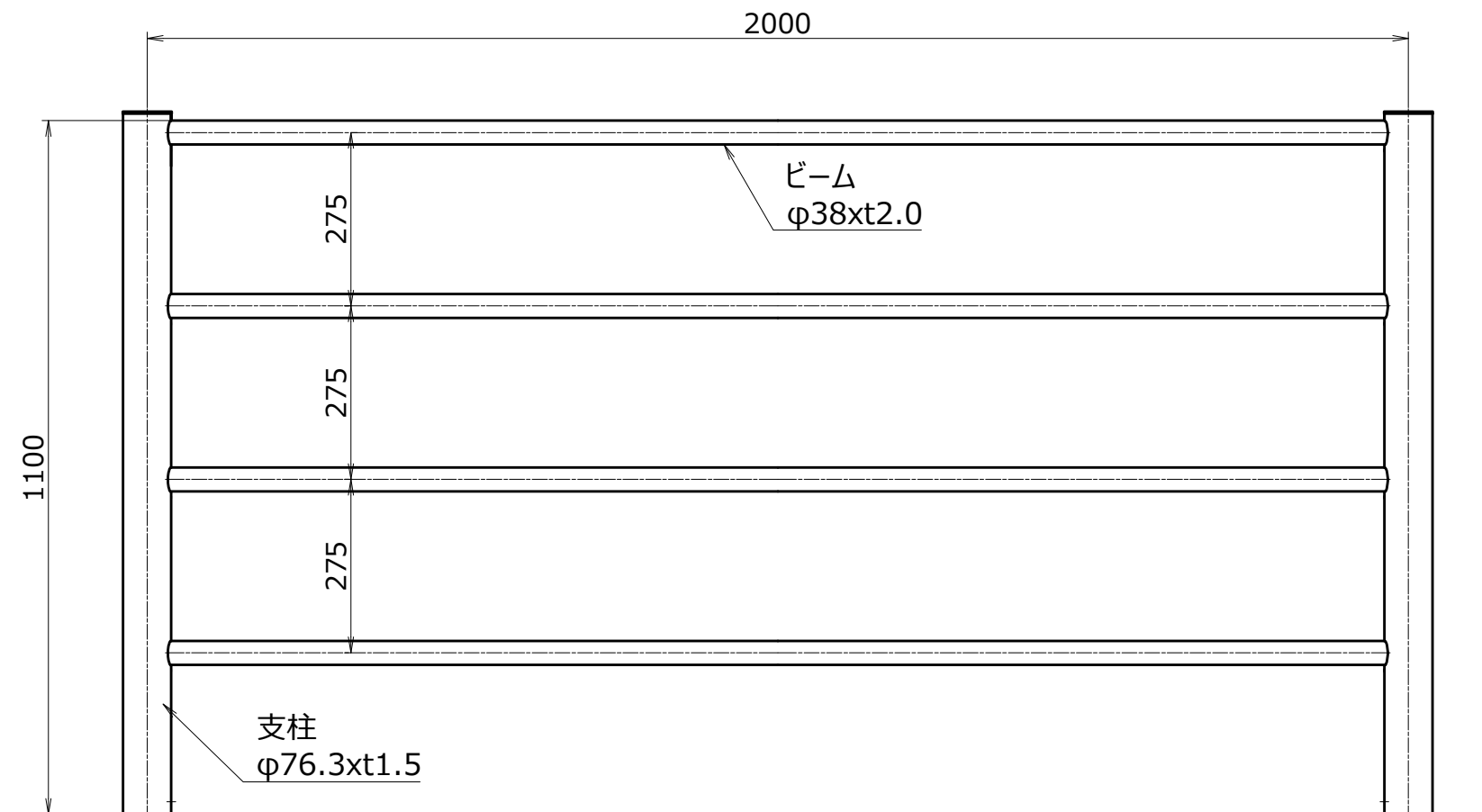
正面図 S=1/10
