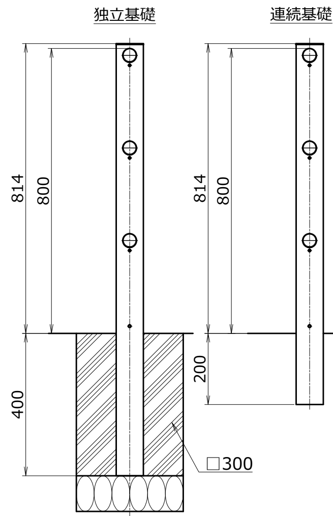
側面図 S=1/10
