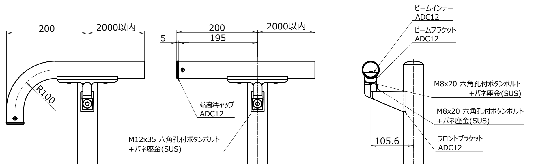
取付詳細図 S=1/5
