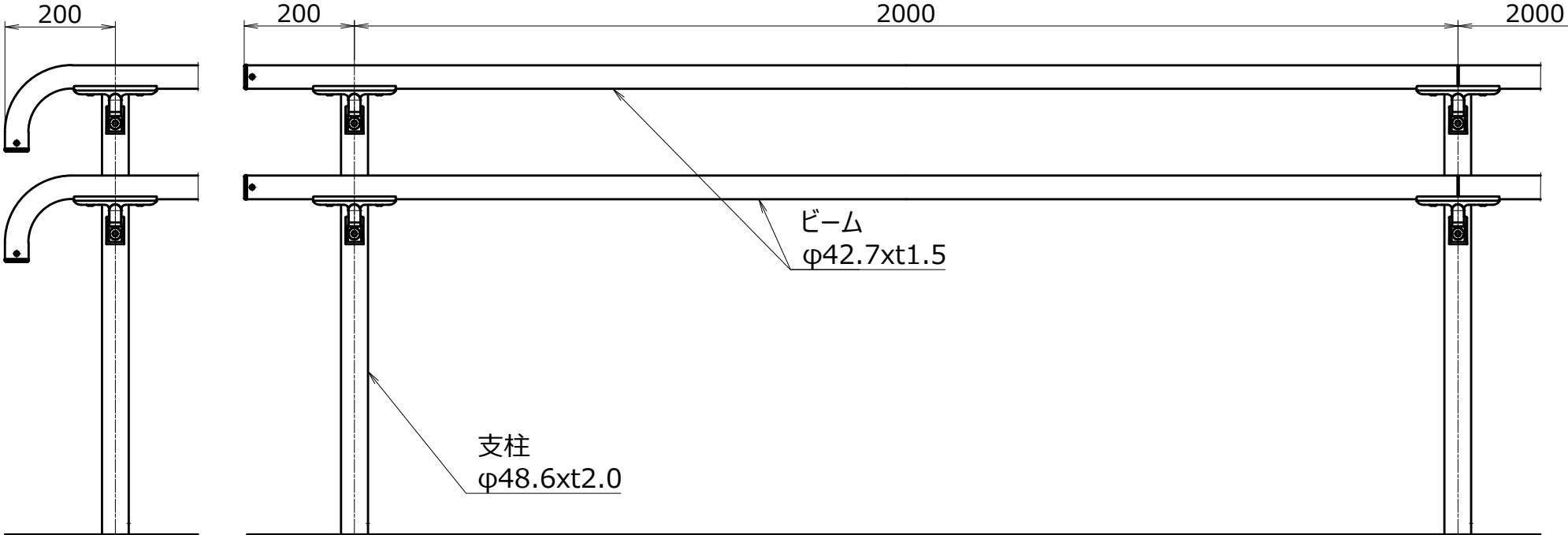
正面図 S=1/10
