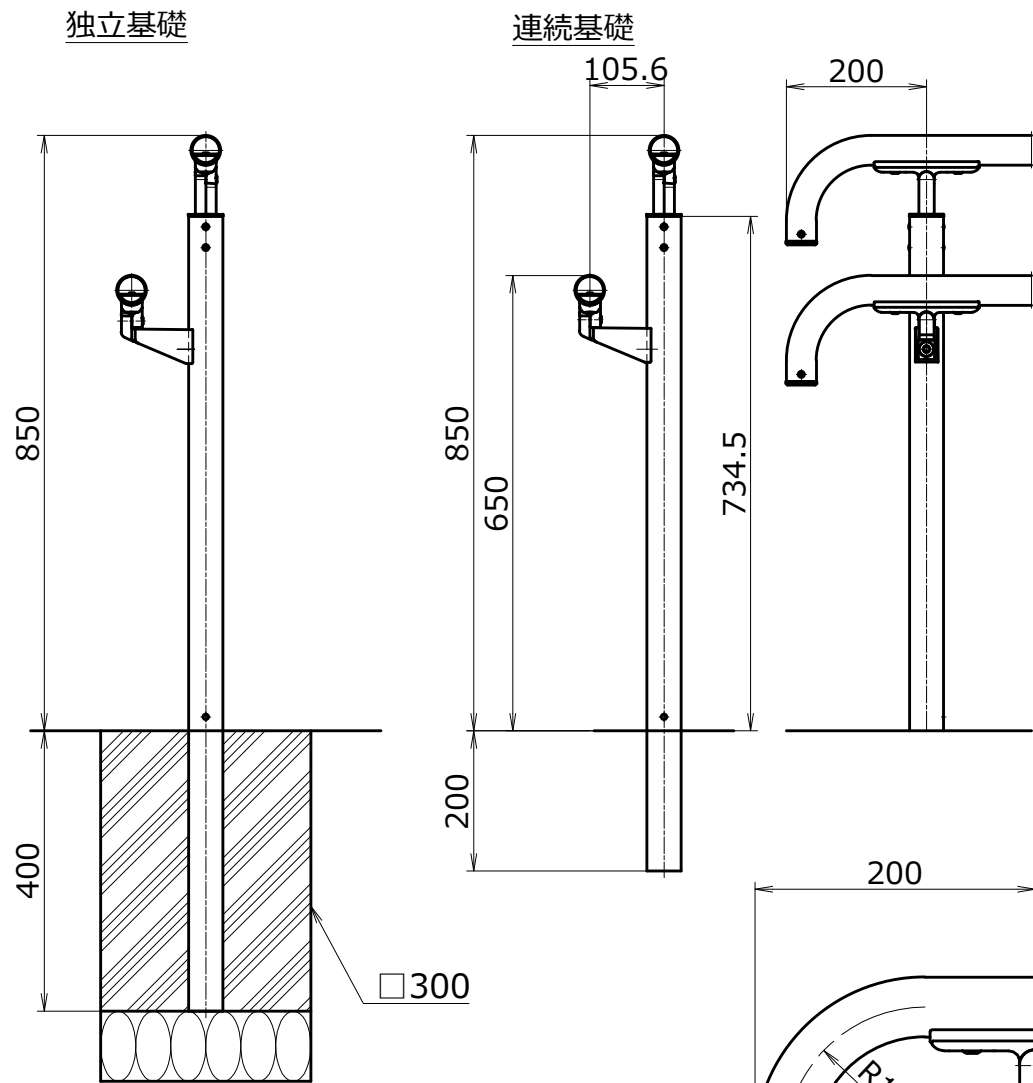
側面図 S=1/10
