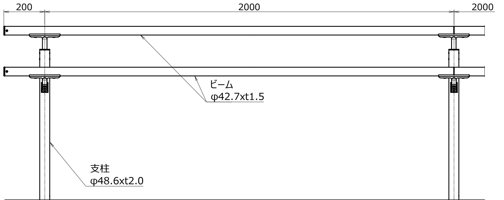
正面図 S=1/10
