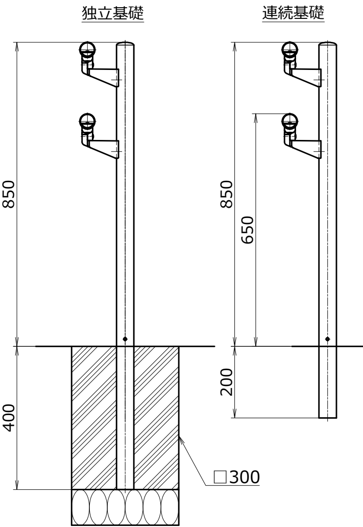
側面図 S=1/10
