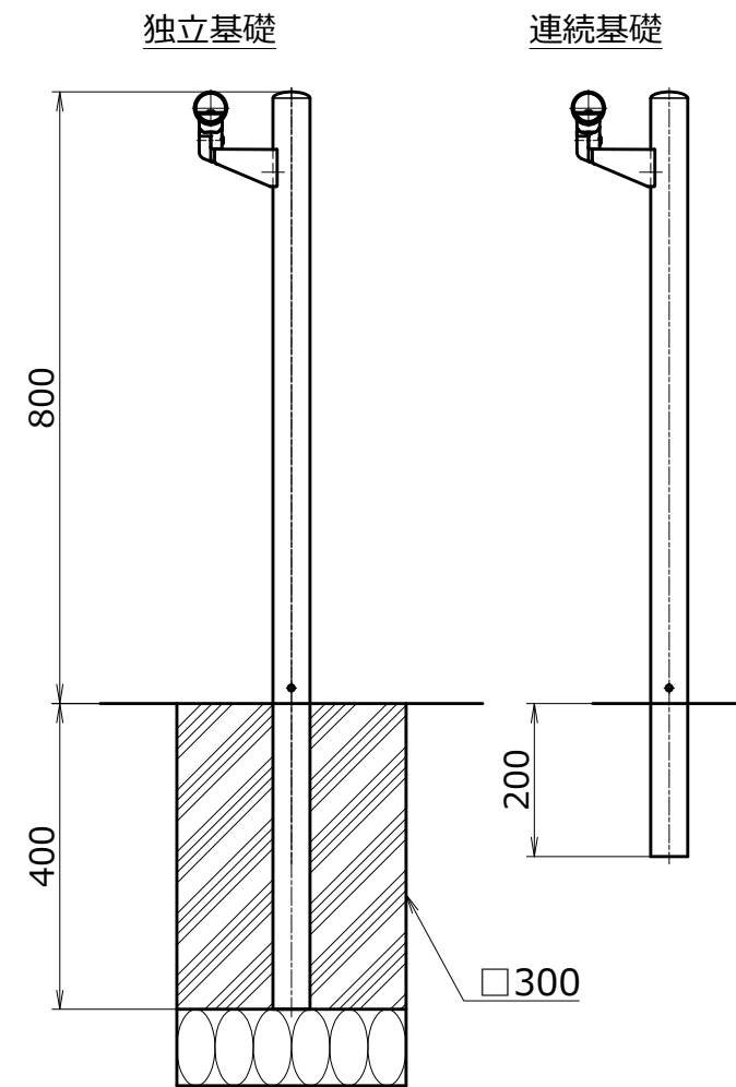
側面図 S=1/10
