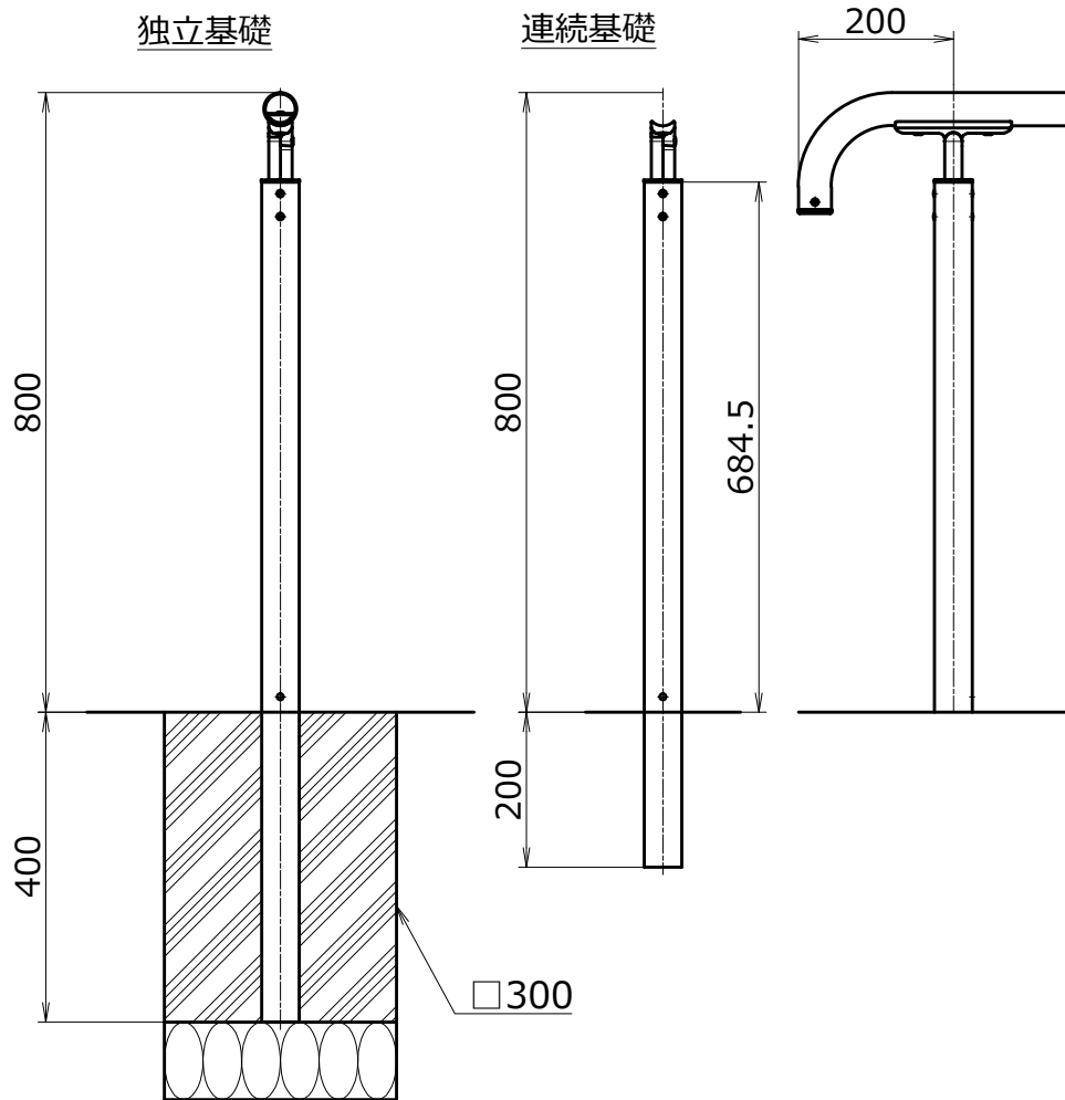
側面図 S=1/10
