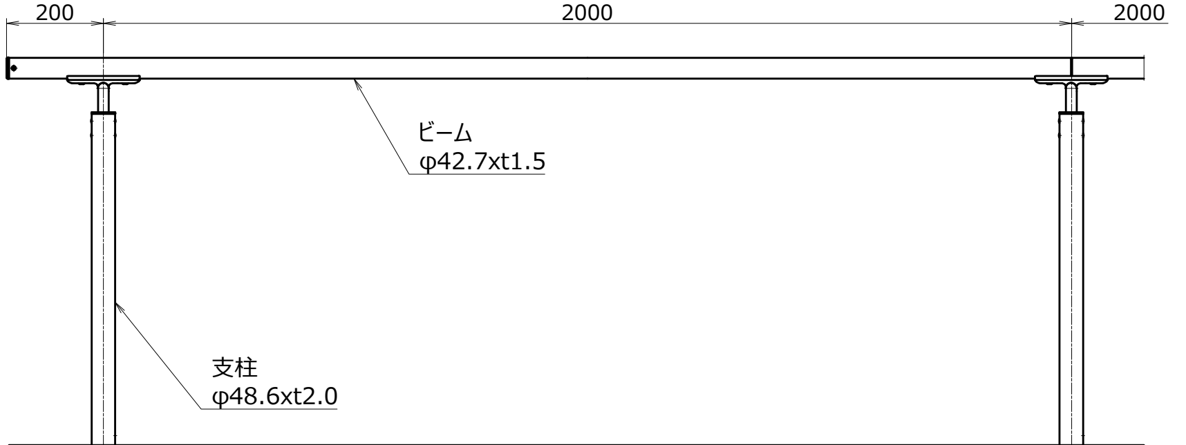
正面図 S=1/10
