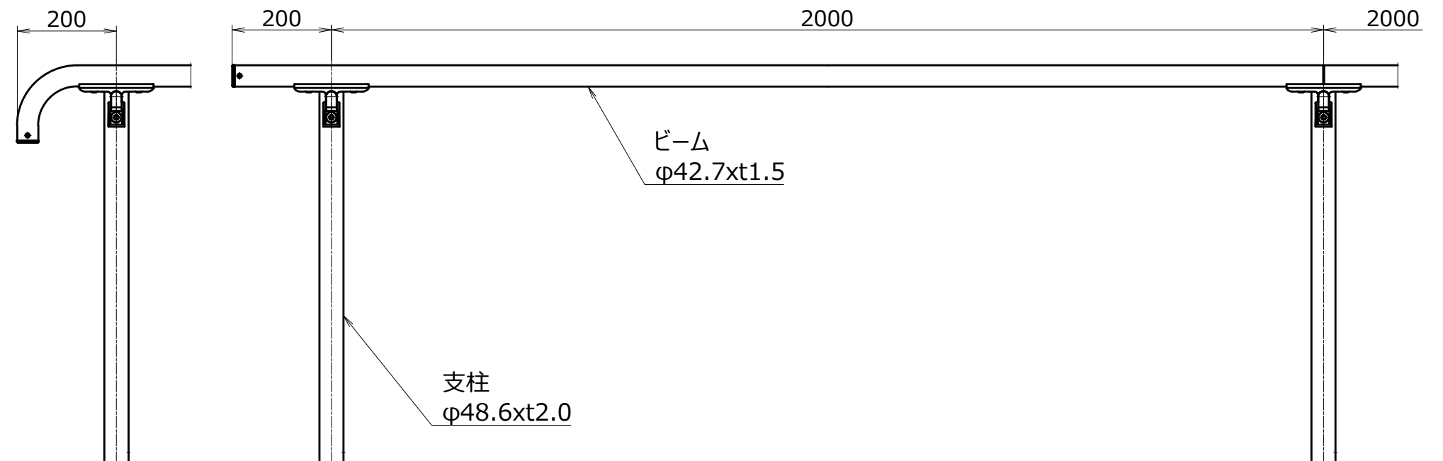
正面図 S=1/10
