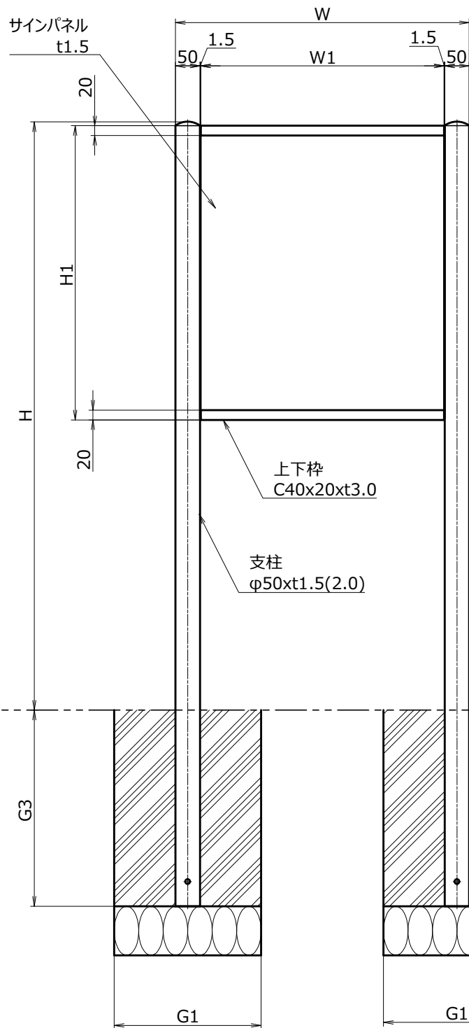
正面図 S=1/10
