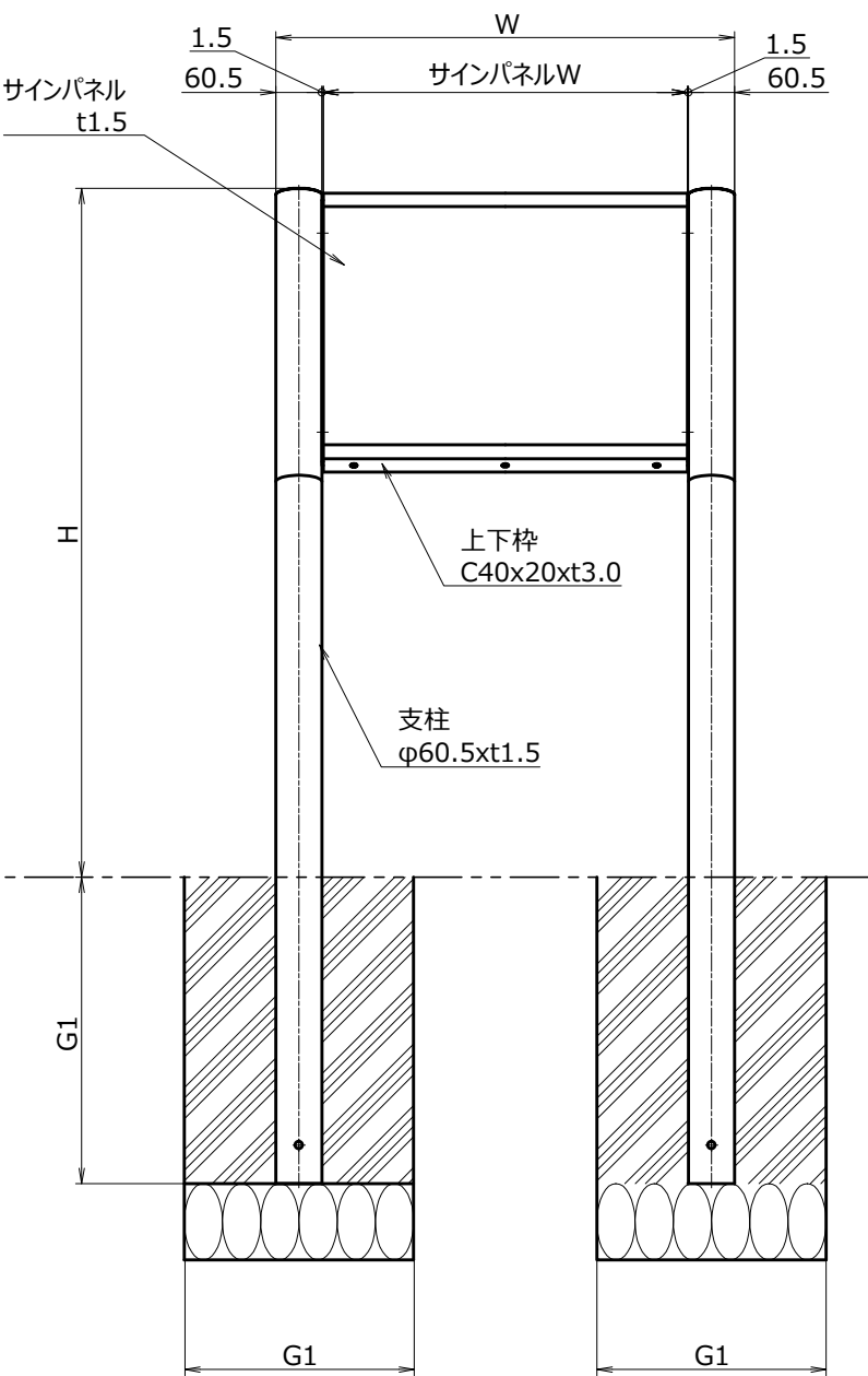
正面図 S=1/10
