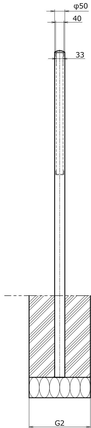
側面図 S=1/10
